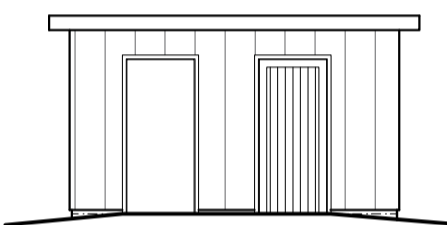
EDRYCHIAD OCHR side elevation 1.100
